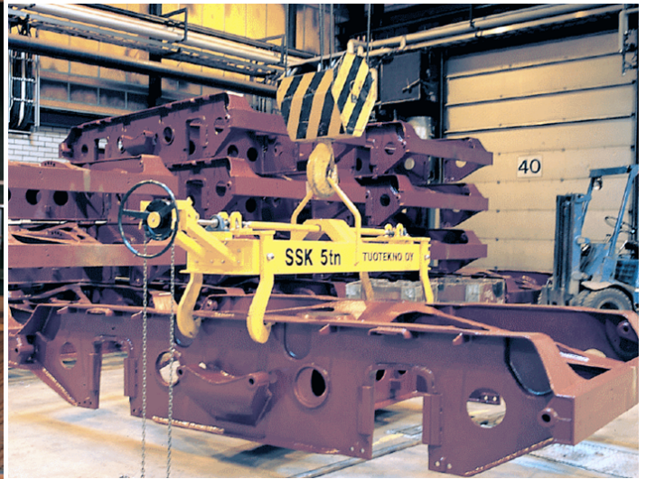
Junatelienn nostoon tarkoitettu nostoapuväline käytössä
