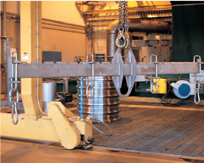
Nosto-orsi haponkestävästä teräksestä elektrolyysikäytössä.
